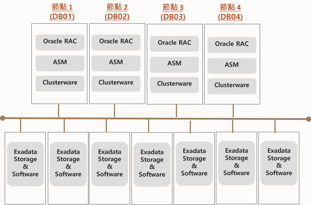
Exadata可橫向擴充資料庫節點
